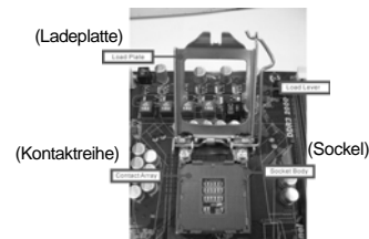
1156-Pin Socket Übersicht
