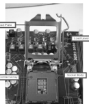
Общий вид 1156-контактного гнезда
